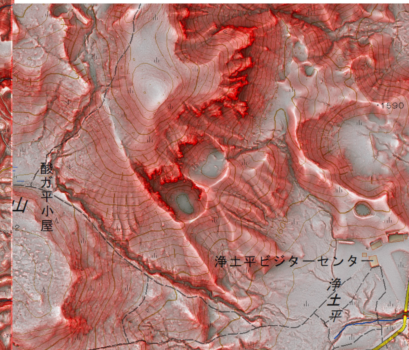
大穴火口周辺の拡大図
